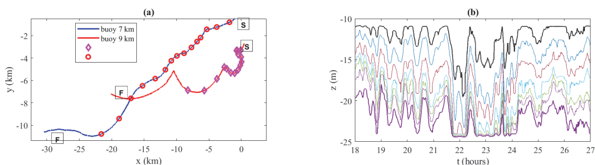
Рис. 1. Регистрация внутренних волн дрейфующими буями с термокосами: (а) траектории дрейфа станций; (б) фрагмент записи деформации изотерм
