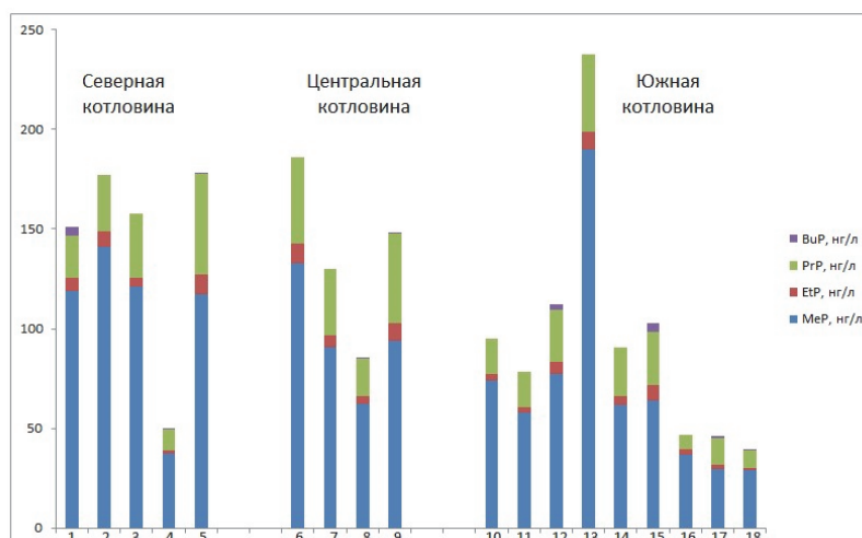
Рис. Суммарная концентрация парабен (нг/л) в воде прибрежной зоны озера: г. Северобайкальск (1), р. Тья (2), пос. Заречный (3), мыс Елохин (4), р. Томпуда (5), пос. Хужир (6), б/о Зуун-Хагун (7), пос. Сахюрта (8), зал. Чивыркуйский (9), бух. Песчаная (10), пос. Листвянка – пос. Танхой (11), пос. Листвянка (12), пос. Маритуй – р. Солзан (13), г. Слюдянка (14), г. Байкальск (15), Байкальск, БЦБК (16), пос. Танхой (17), р. Селенга (18)
