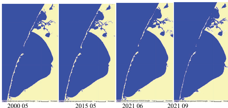
Рис. 2. Сравнение конфигурации береговой линии п-ова Карга по сезонам
