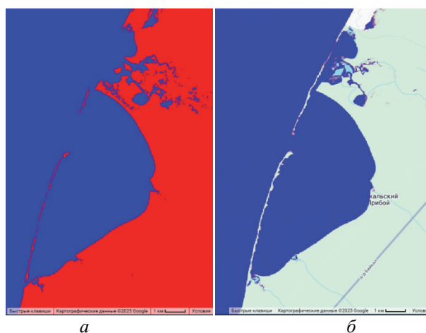
Рис. 3. Стабильные участки территории (а) и максимально возможная территория (б) п-ова Карга
