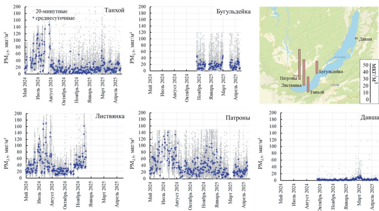
Рис. Карта расположения станций и измерения PM_{2.5} на станциях Танхой, Листвянка, Бугульдейка, Патроны, Давша. Серыми точками обозначены 20-минутные концентрации PM_{2.5} , синими – среднесуточные, красными – медианные концентрации
