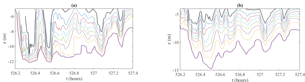
Рис. 2. Эволюция изотерм на двух автономных станциях, расположенных на глубине 13 м (a) и 34 м (b)
