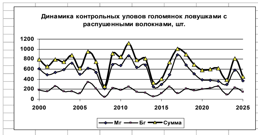
Рис. 1. Динамика уловов голомянковыми ловушками за последние 25 лет
