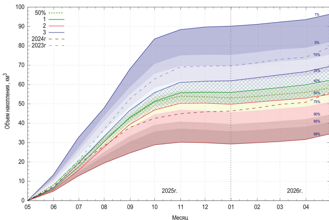
Рис. Пример отображения области расположения прогнозируемых гидрографов интегрального полезного притока в оз. Байкал: вероятная (1), нижняя (2), верхняя (3) прогностические границы
