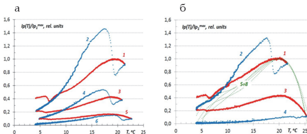
Рис. Зависимость интенсивности свечения воды р. Ангарты от температуры.
