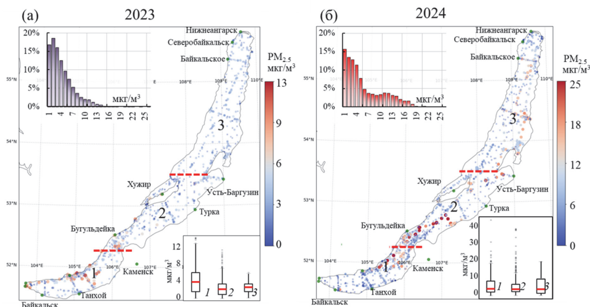
Рис. Пространственное распространение среднечасовых концентраций PM_{2.5} : (а) с 17 июня по 1 ноября 2023 г. ; (б) с 30 мая по 20 октября 2024 г.
