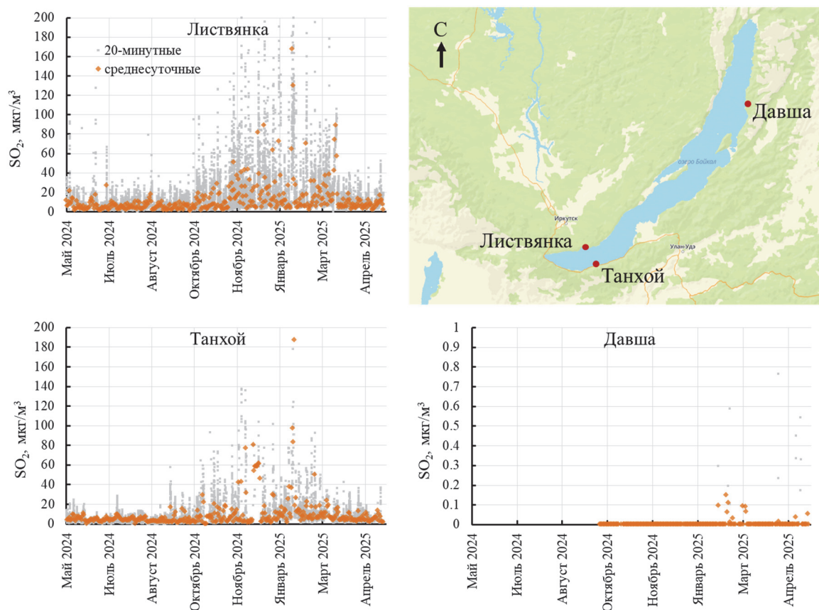
Рис. Результаты автоматического мониторинга SO 2 в приземном слое атмосферы в ЦЭЗ Байкала, 2024–2025 гг.
