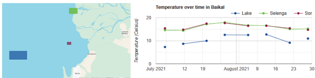
Рис. 3. Пример оценки температуры поверхности по трем выбранным участкам
