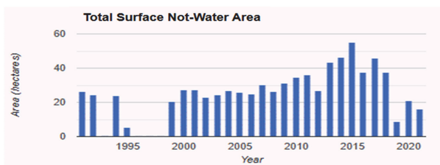
Рис. 1. Зона интереса и колебания площади полуострова Карга оз. Байкал
