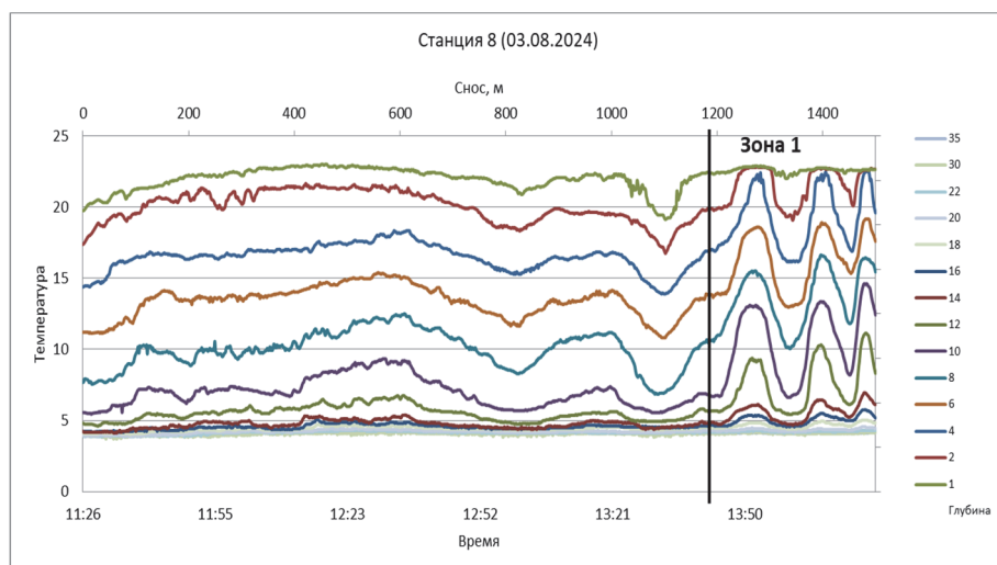
Рис. Временная стратификация температуры в Камгинском заливе с интервалом по глубине 1 м (от 03.08.2024)
