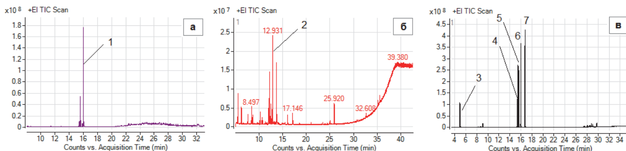
Рис. 1. Хроматограммы продуктов алкилирования бензола: 1 – 2-хлордекан, 2 – 2-децилбензол, 3 – децен-1, 4–7 – изомеры линейного децилбензола
