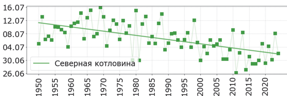
Рис. Динамика достижения температуры воды 4 °C в Дагарской губе (северная котловина оз. Байкал)
